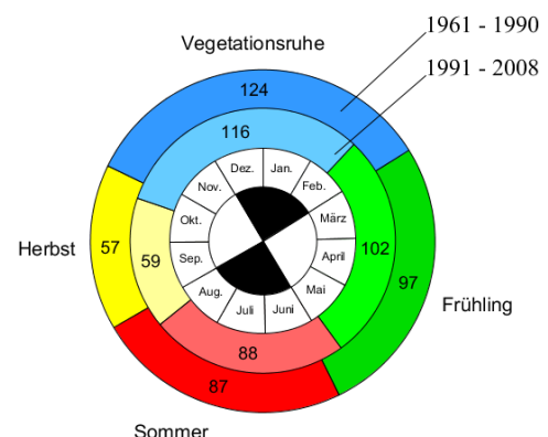
Vereinfachte doppelte phänologische Uhr mit beobachteten mittleren Eintrittsterminen für Hessen (vgl. Tabelle Seite 3)
